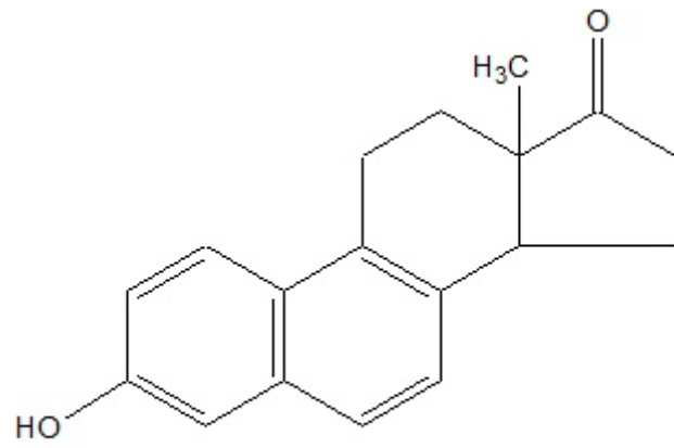
Equilenin
